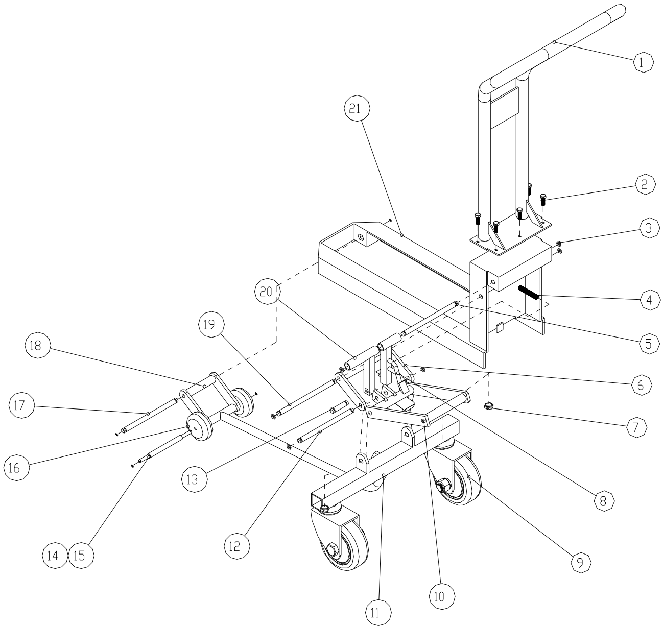
Abbildung 1 Explosionszeichnung
