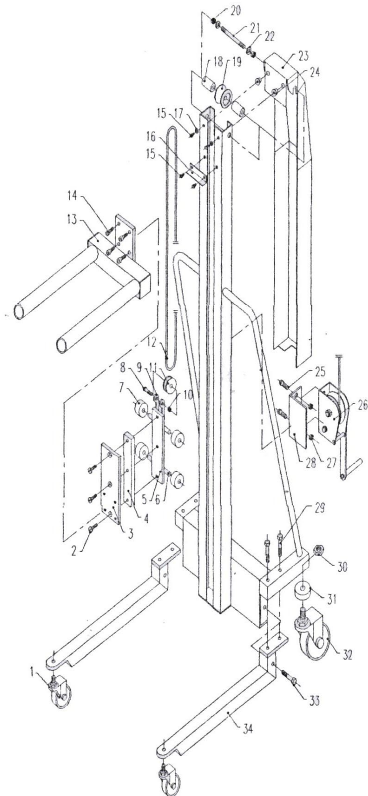
Abbildung 1 Rahmen MES100-15-05
