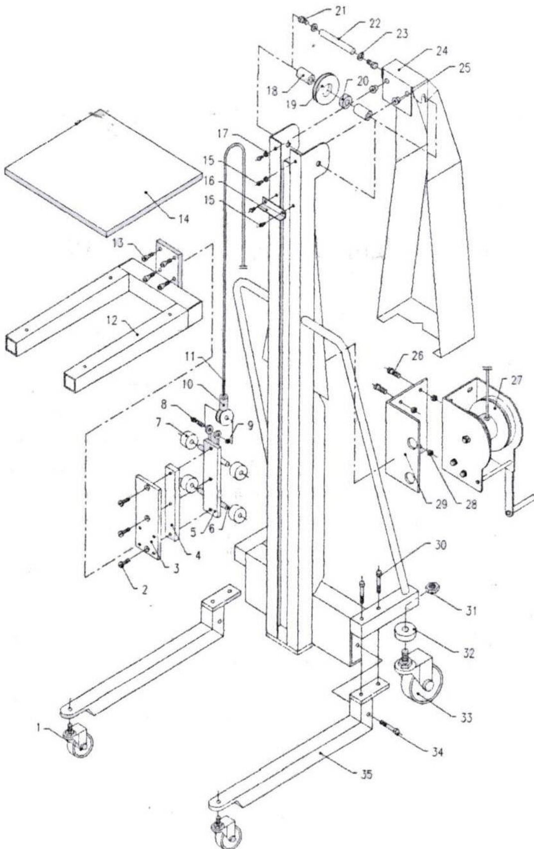
Abbildung 3 Rahmen MES200-15-05
