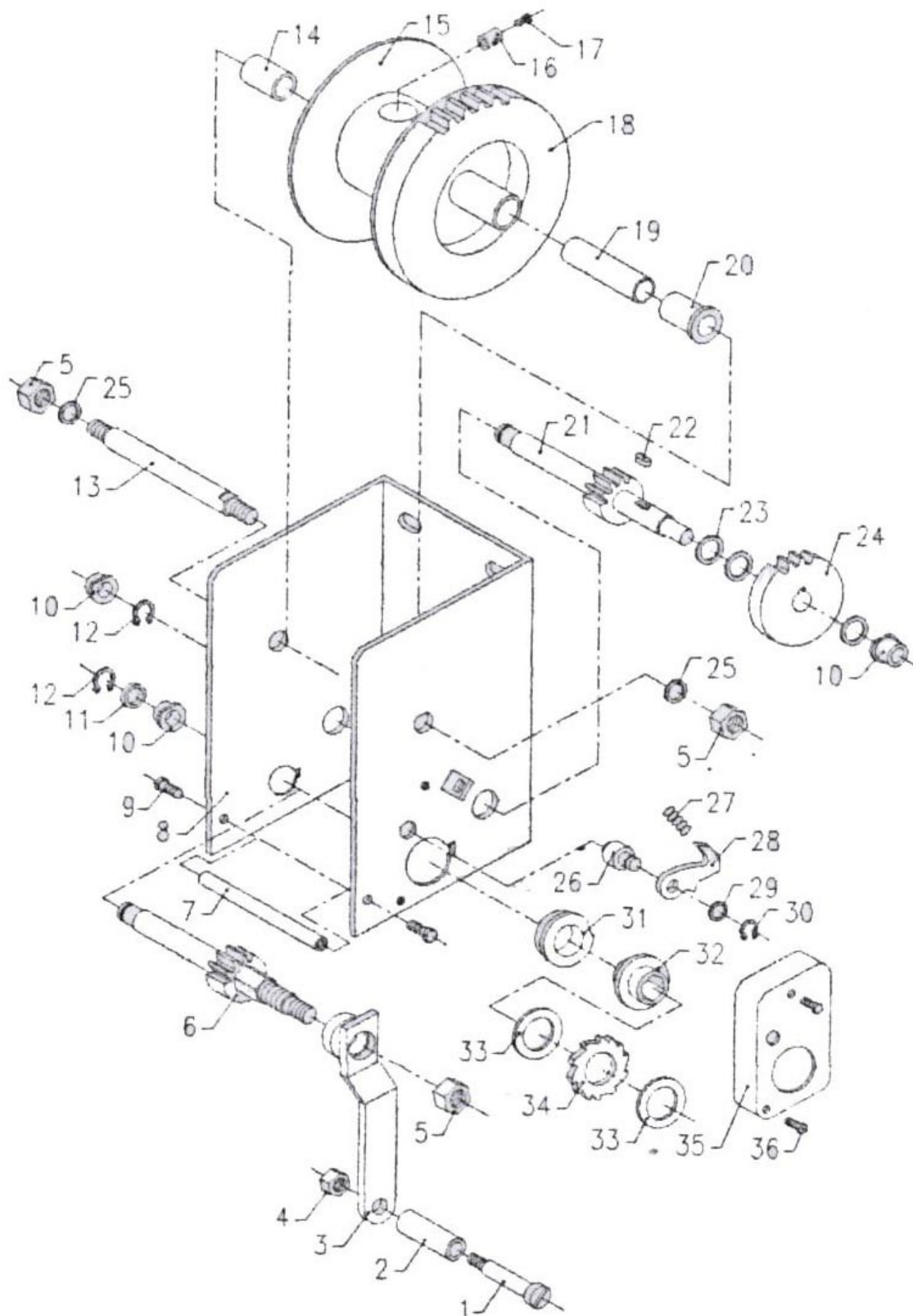
Abbildung 4 Seilwinde MES200-15-05
