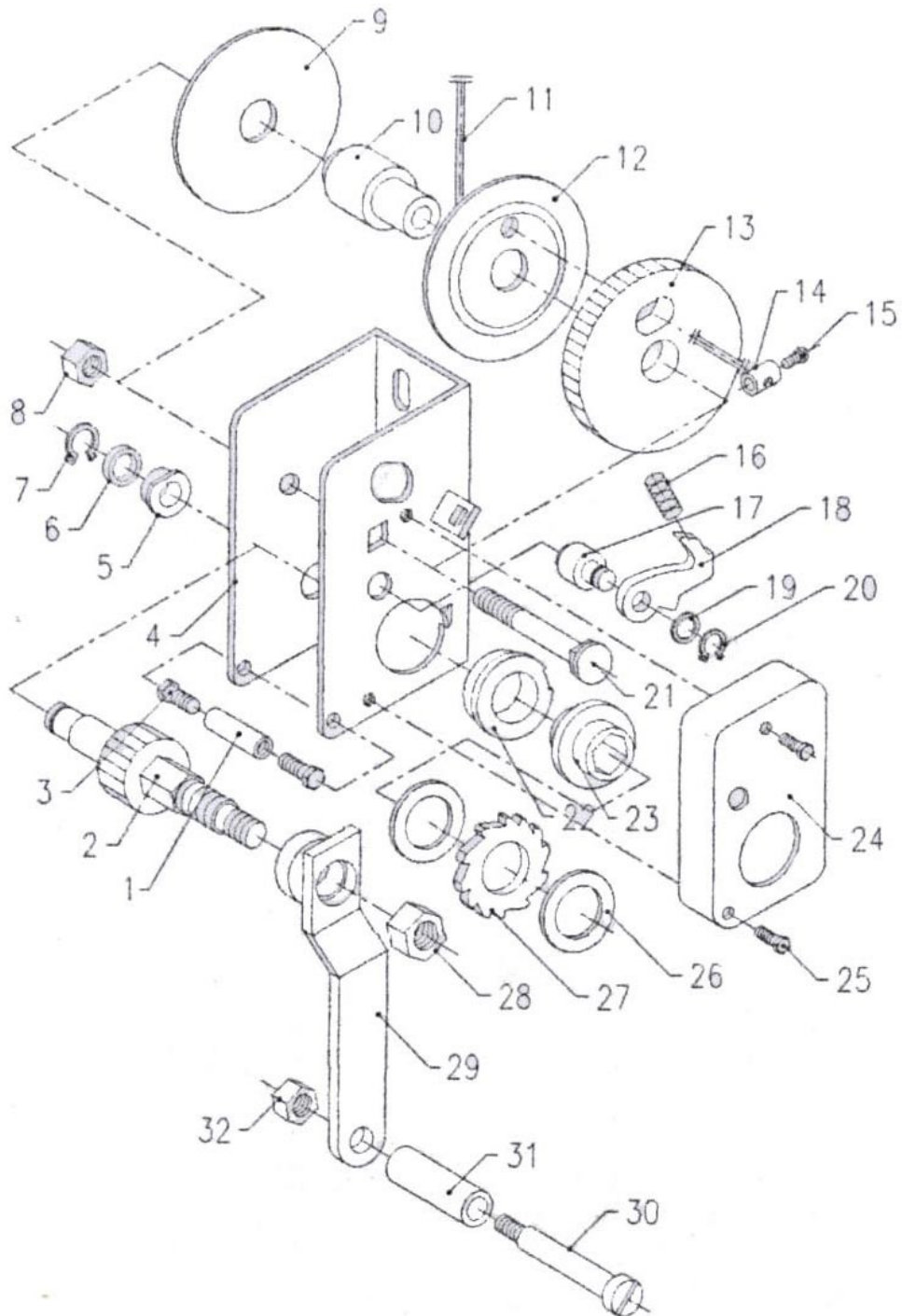
Abbildung 2 Seilwinde MES100-15-05
